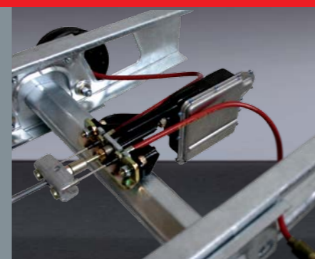
Система контроля прицепа АТС
