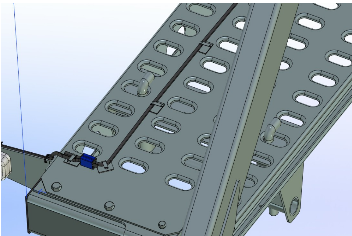
Рисунок 12. Упор колёсный, вид снизу.
