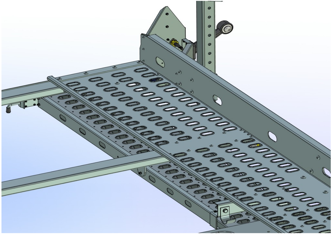
Рисунок 9 - Трап в транспортном положении
