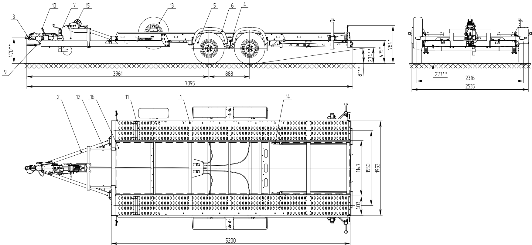
Рисунок 1 - Прицеп МЗСА 852131 (исполнение 301).
