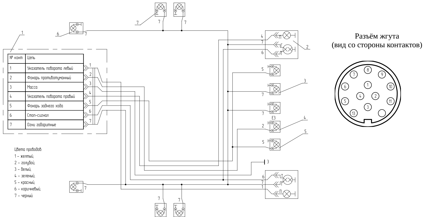
Рисунок 2 – Схема электрооборудования
